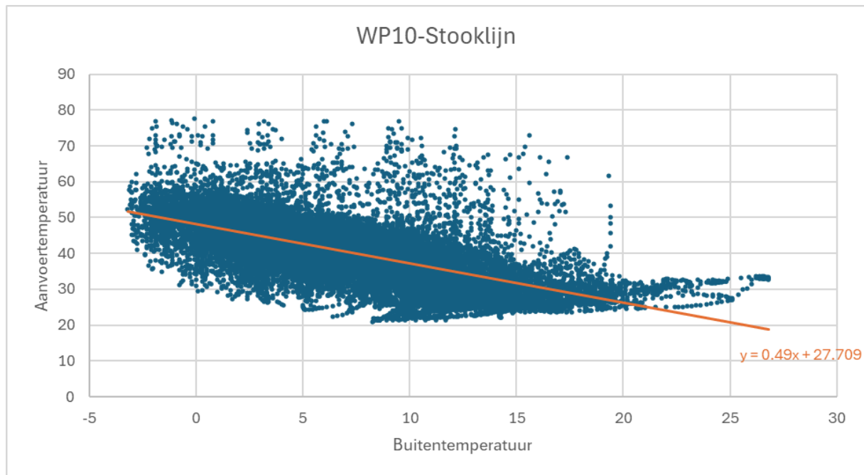
Figuur 3: Stooklijnen
