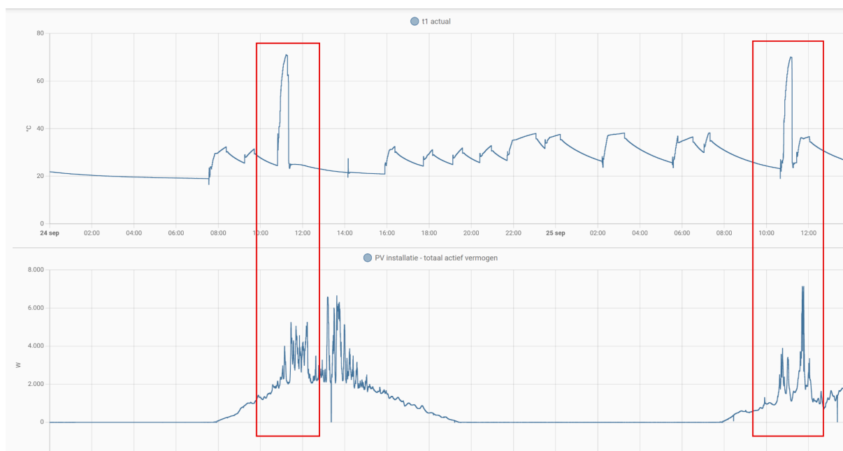
Figuur 18: Aanvoertemperatuur versus opbrengst PV-installatie bij WP7
