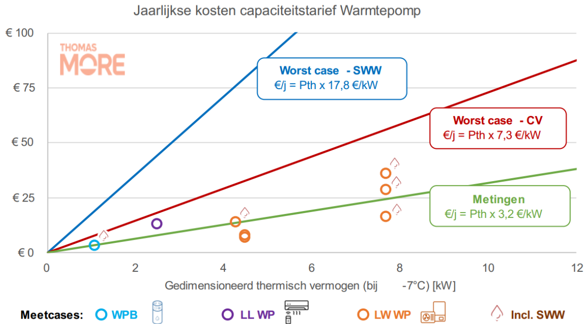
Figuur 15: Invloed van een warmtepomp op het capaciteitsstarief (Thermi-Var)
