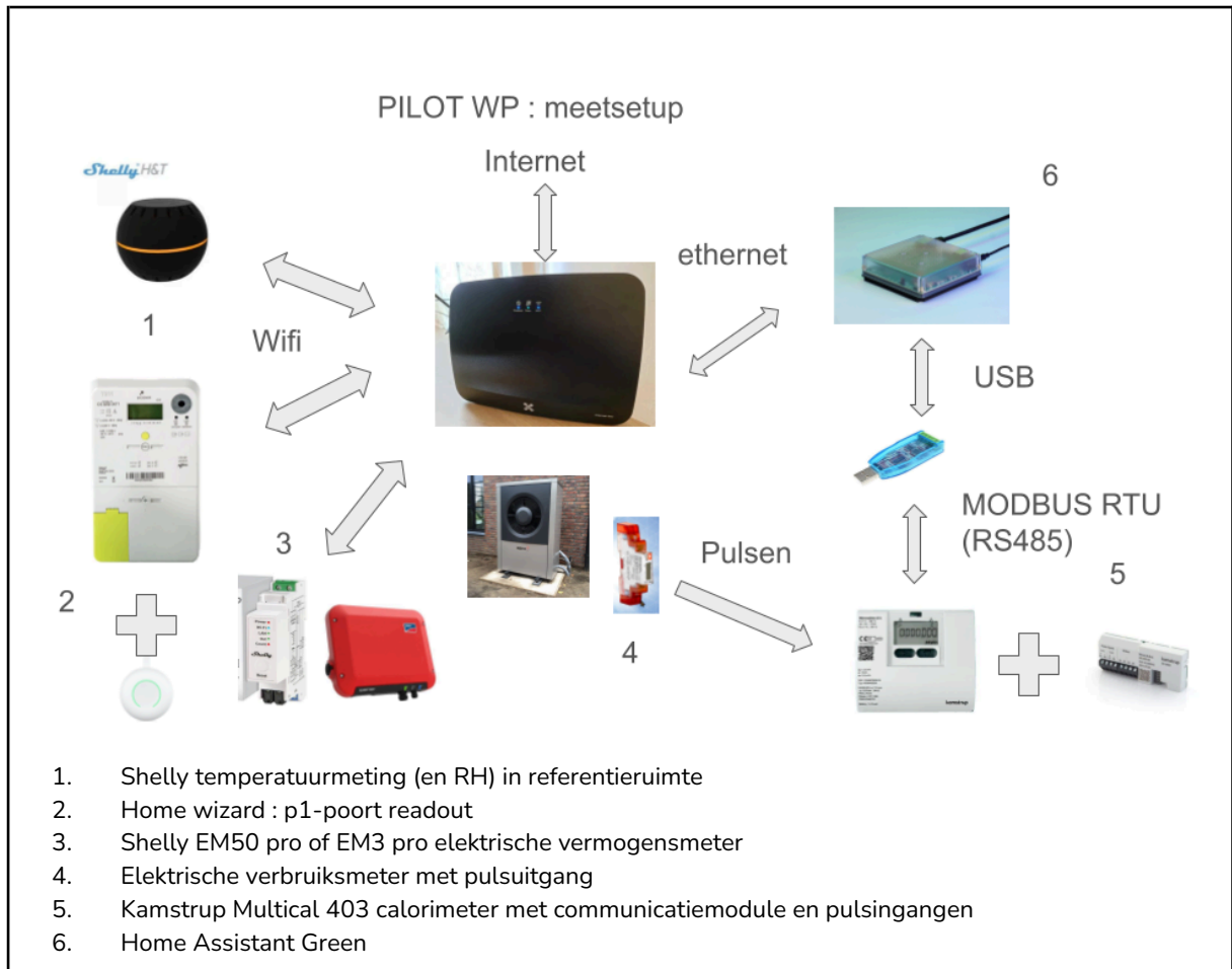
Figuur 1: Meetopstelling
